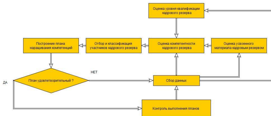
Приложение Д. Рис.17. Алгоритм построения плана наращивания компетенций
