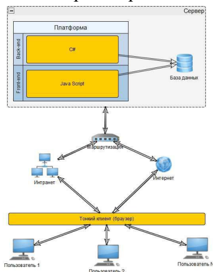
Приложение Д. Рис. 29. Архитектура Web –приложения СПКР.
