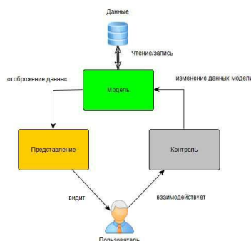
Приложение Д. Рис. 30. Структура MVC - шаблона.
