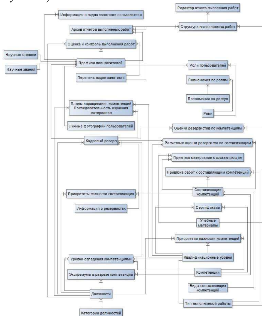
Приложение Д. Рис. 31. Реляционная структура базы данных СПКР.
